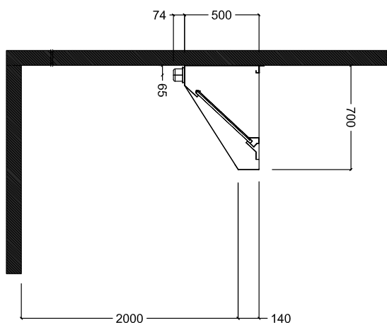
Вид сбоку
